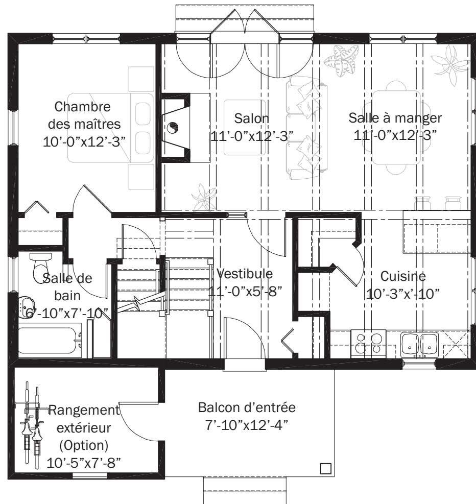
Plan du rez-de-chaussée 24'-0" x 32'-0" 816 pi.ca.
