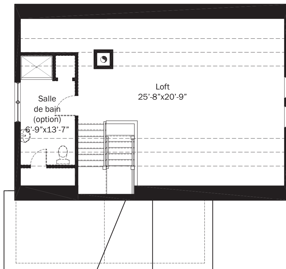
Plan de l'étage 24'-0" x 32'-0" 816 pi.ca.
